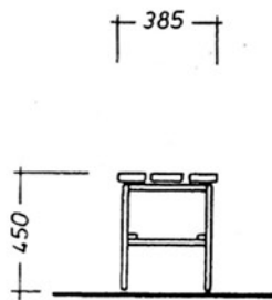
Sitzbank als freistehende Hockerbankkonstruktion.
