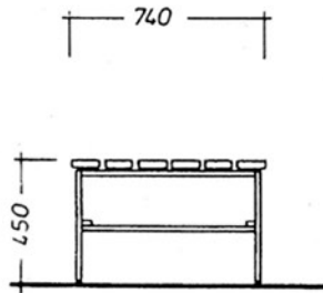
Doppelsitzbank als freistehende Hockerbankkonstruktion.
