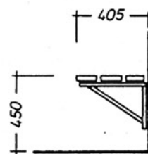
Fußfreie Sitzbank mit Wandbefestigung.
