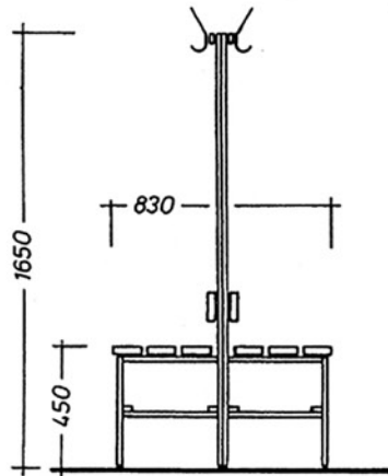
Doppelseitige Sitzbank mit Hakenleiste und Rückenlehne.
