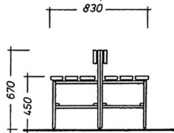
Doppelseitige Sitzbank mit niedriger Rückenlehne.
