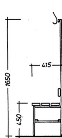
Einseitige Sitzbank mit Hakenleiste und Rückenlehne.
