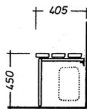
Sitzbank mit vorderem Stützfuß und Wandbefestigung.
